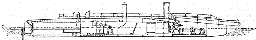
Миноноска 163
