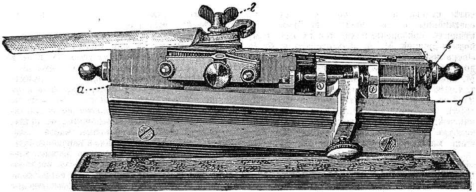
М. протомъ (одна изъ простѣйшихъ конструкцій): а—подставка, въ которой укрѣпится на пробѣ разрывае-мый, завитый объектъ; б—вазъ-никая плоскость, по которой, съ помощью микрометрическаго винта (с), движется подставка; в—рычагъ для прикрѣпления брызговъ (ср) къ подставкѣ, движущейся горизонтально. Одна изъ такъ наз. санпыхъ микрономовъ (Schlittemikrotom).
