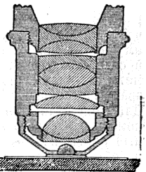
Фиг. 4. Апохроматъ Цейсса съ однородной иммерзіей.
