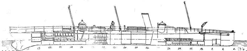
1. Миносец типа Шиху.
