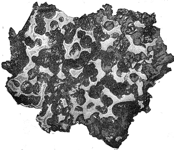
Палласово желѣзо.
